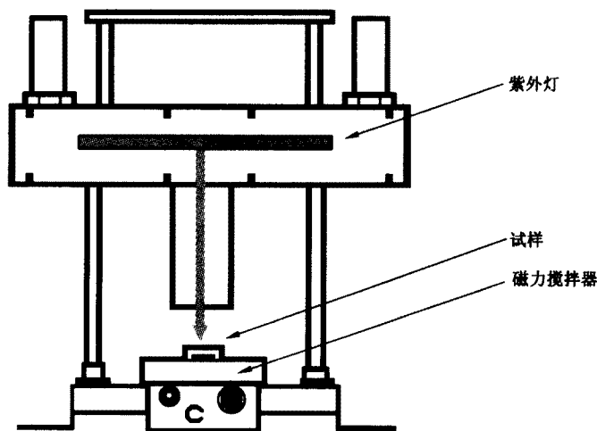
图 D.1 平行光束测试示意图
